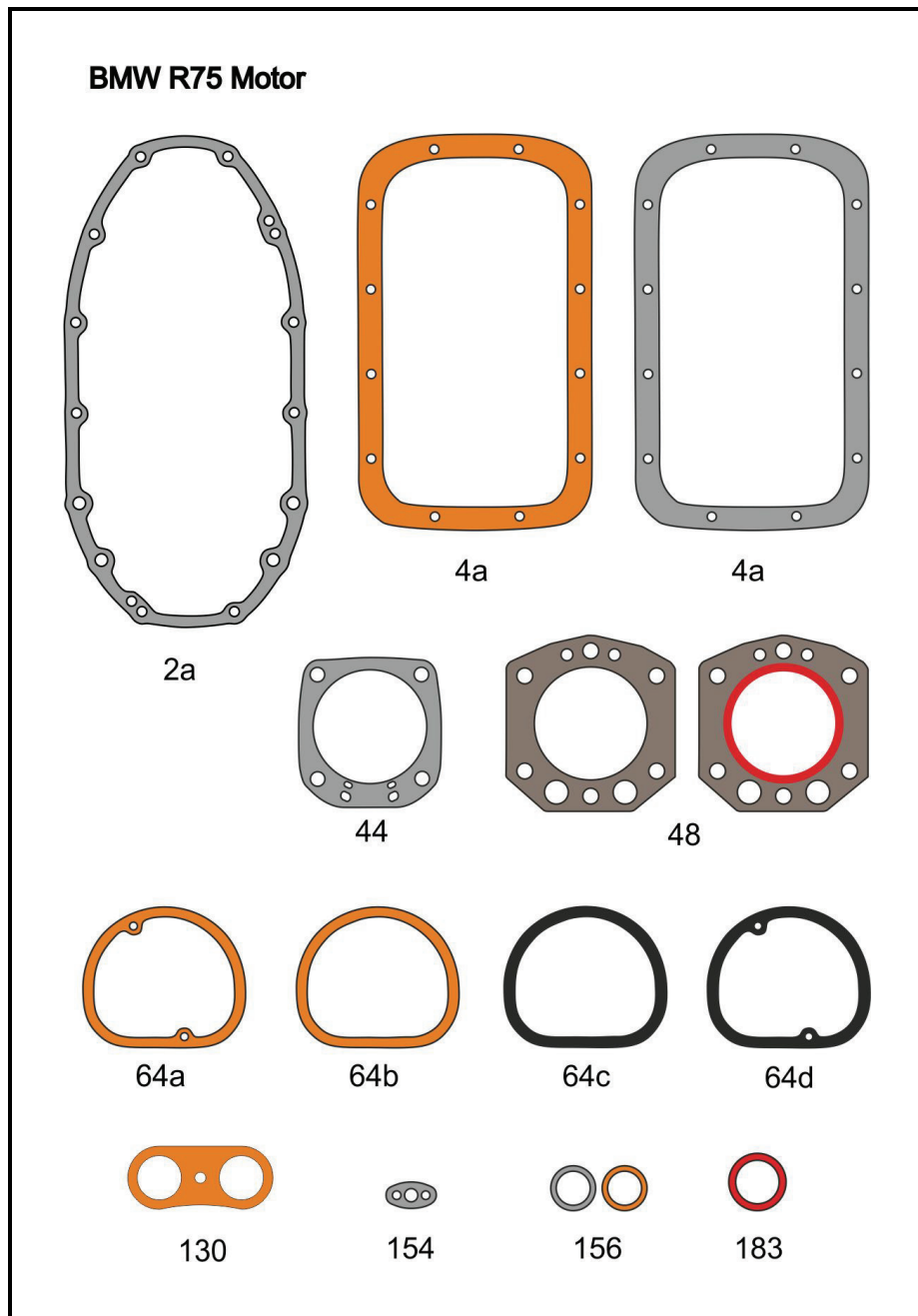
Tafel 50: Dichtungen BMW R75 Motor
