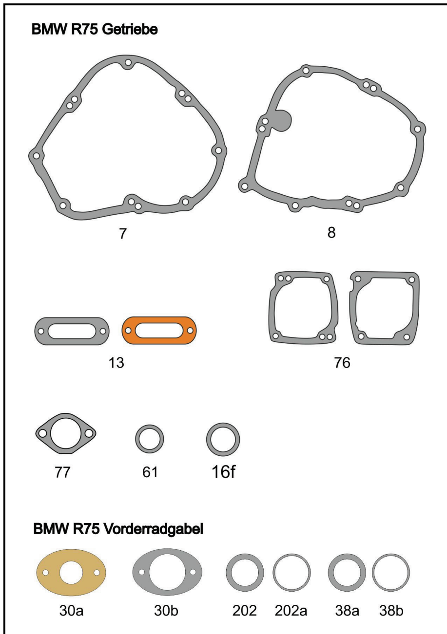
Tafel 51: Dichtungen BMW R75
